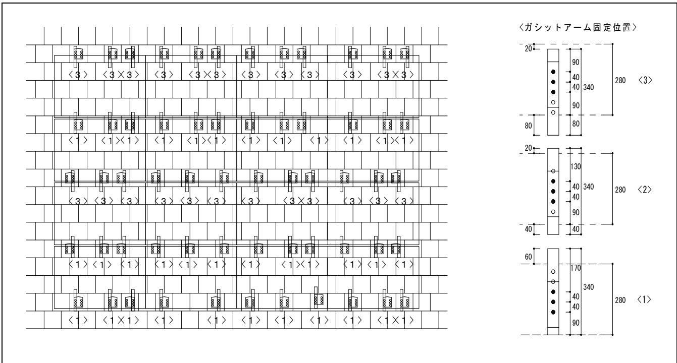
PV 支持金具納まり図
