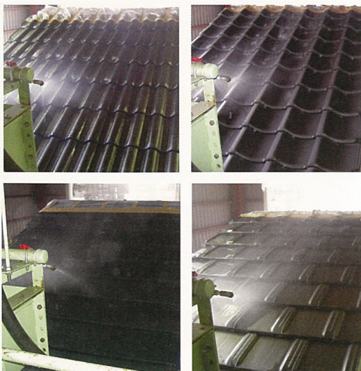
最大風速60m/s・雨量200mm/hの条件で室内側への漏水無しを目視確認。
