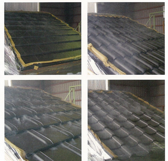
発煙筒にて小屋裏に煙を発生させ、瓦の隙間等からの排煙状況を確認。
