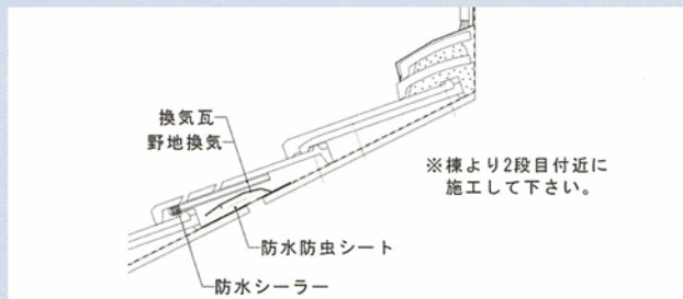
下屋根・壁際部取付け納まり図
