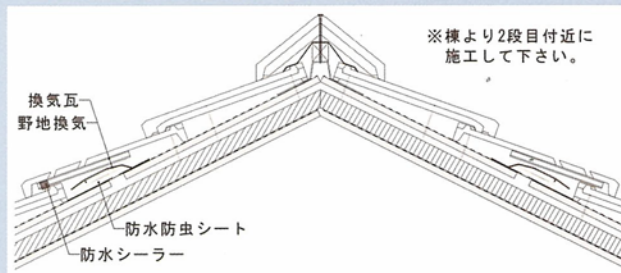
屋根断熱通気・大棟部取付け納まり図
