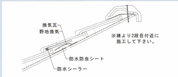
屋根断熱通気・大棟部取付け納まり図
